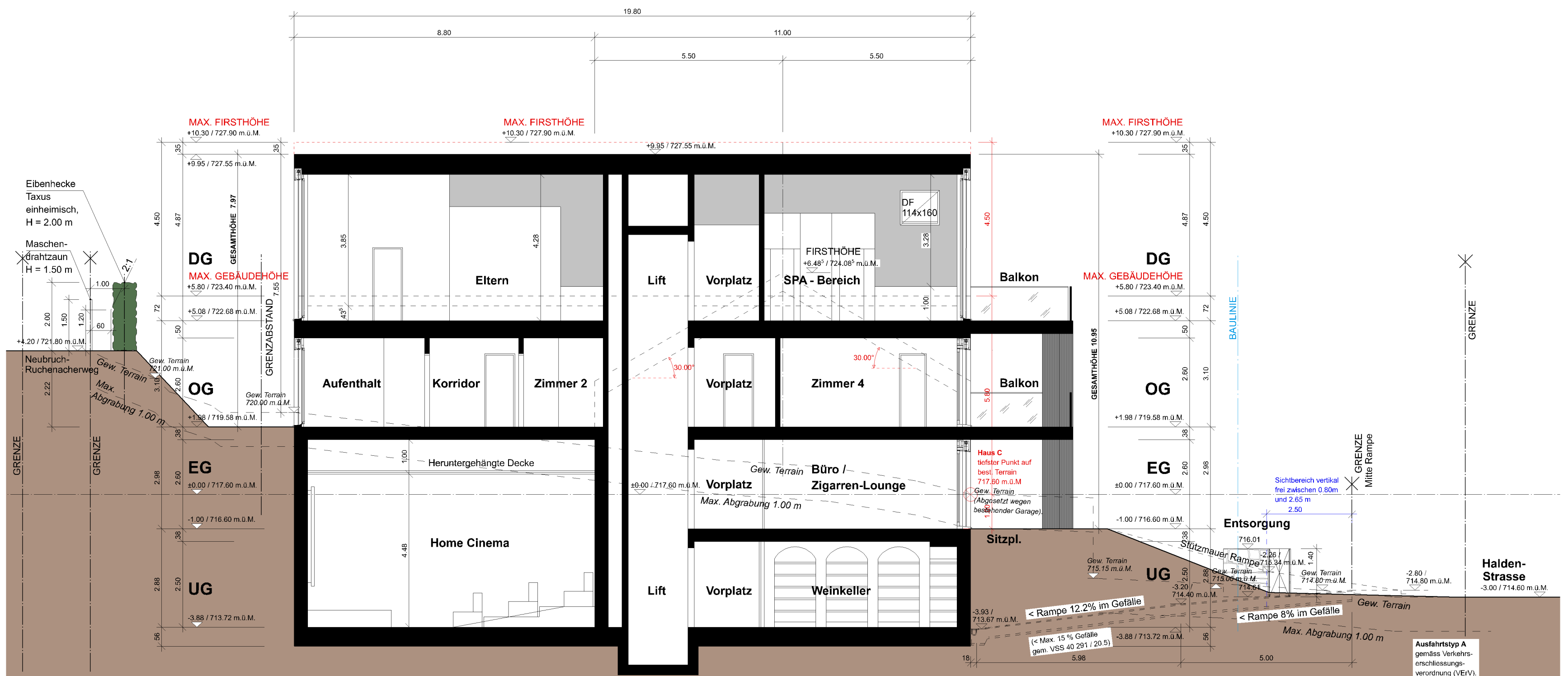
SC2 - Schnitt Haus C
