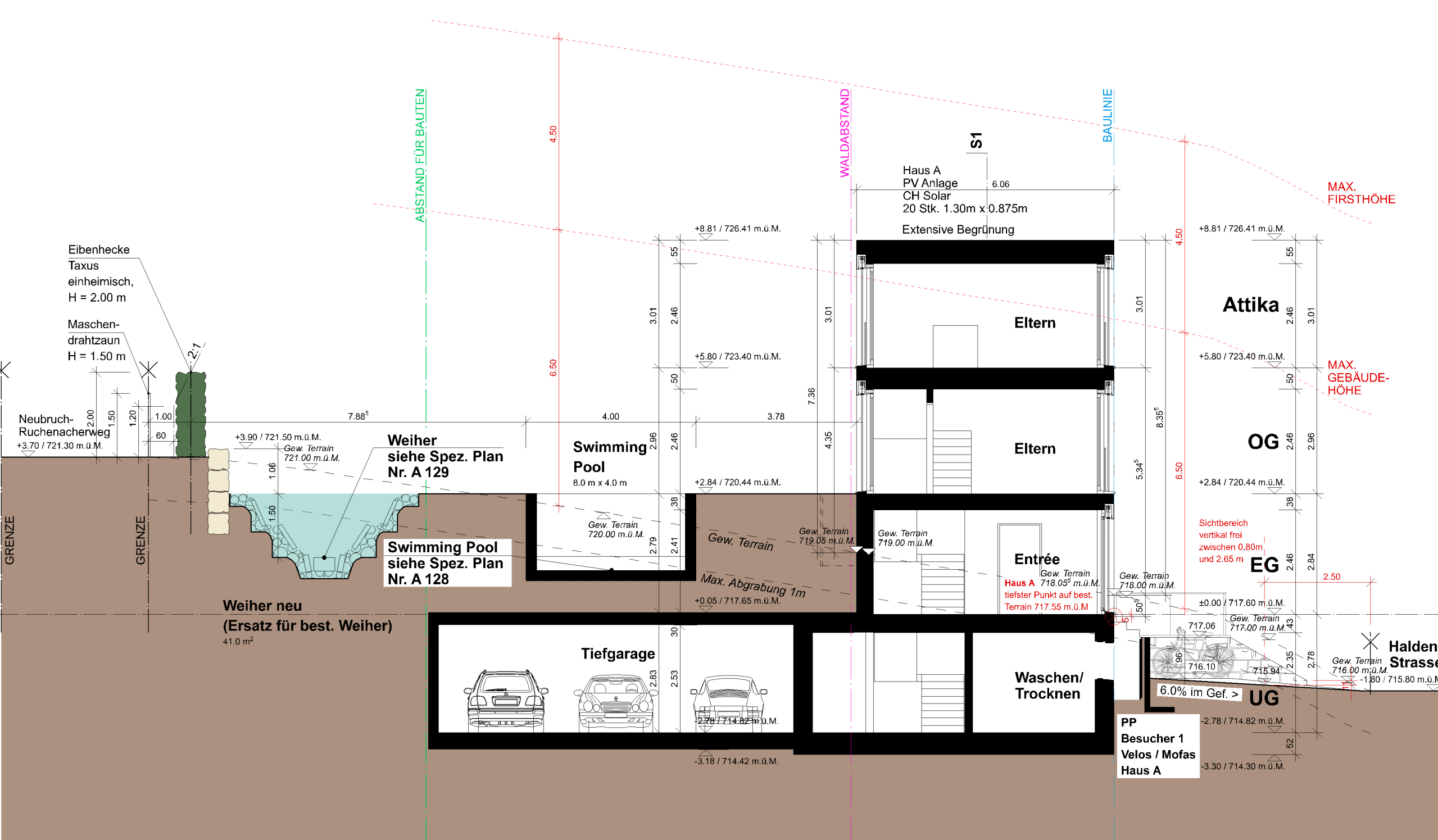
SA1 - Schnitt Haus A
