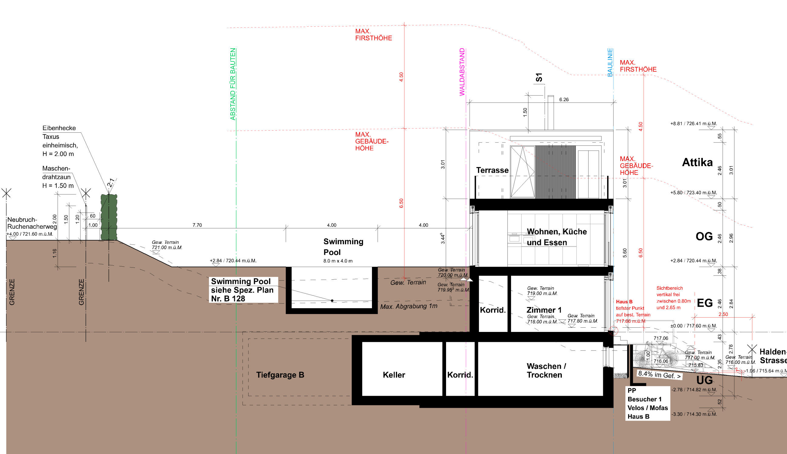
SB1 - Schnitt Haus B
